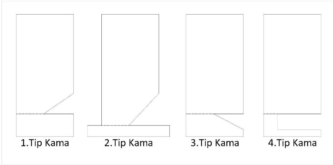
Şekil 2.15 Kama şekilleri
